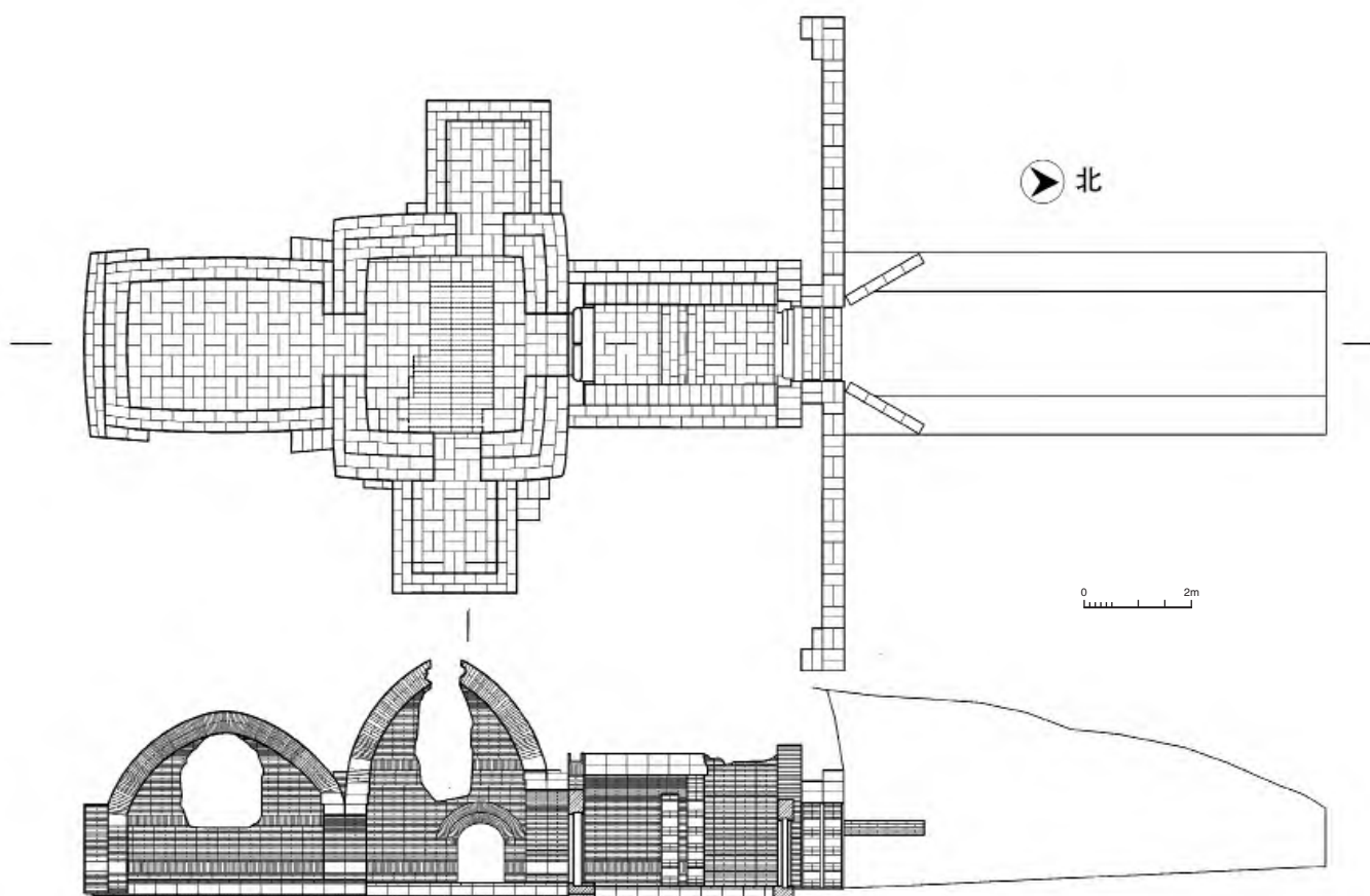
M1 平剖面
